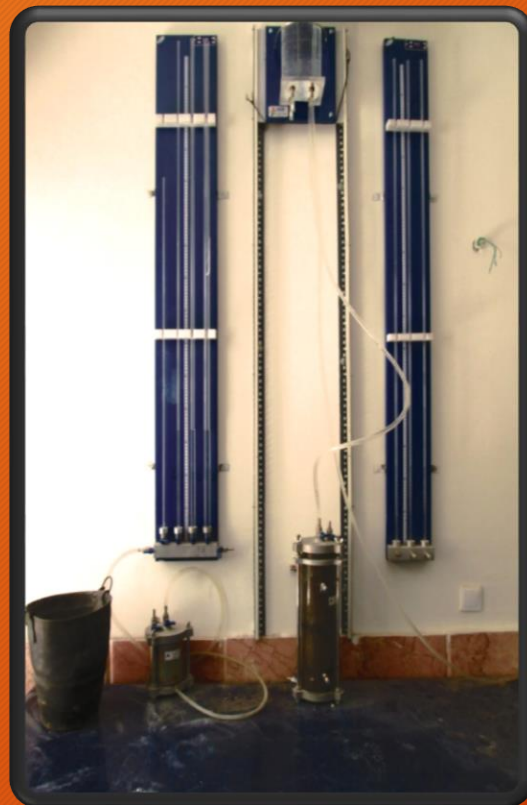
دستگاه نفوذ پذیری
